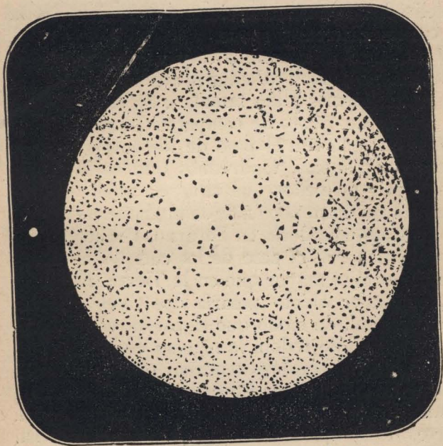
El Sol: tamaño aparente visto desde la Tierra y desde N.º p'uno.
